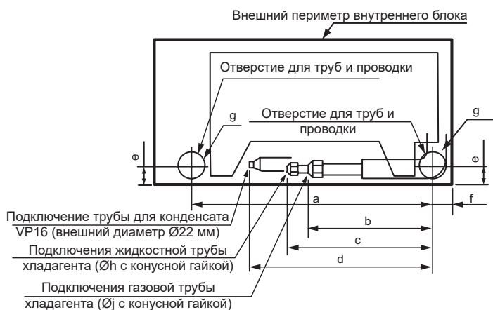
Вид внутреннего блока спереди
